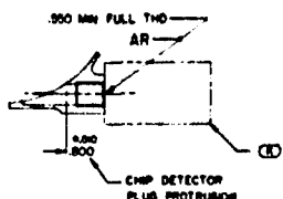
TYP CMP DETECTOR OTHER LOC (D)
